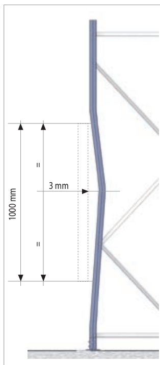
A) Prehnuté stĺpy v smere roviny rámu, s trvalou deformáciou rovnou alebo väčšou než 3 mm, zmeranou v strede úseku „a“ s dĺžkou 1 m.
