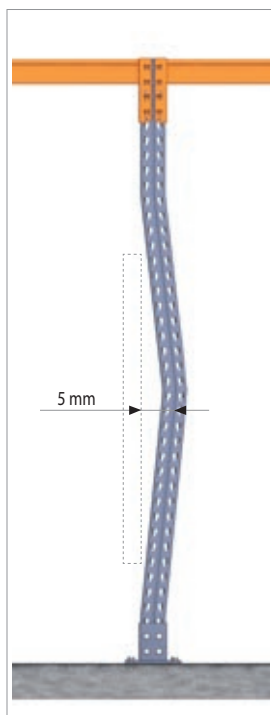
B) Prehnuté stĺpy v smere roviny nosných trámov, s trvalou deformáciou rovnou alebo väčšou než 5 mm, zmeranou v strede úseku „a“ s dĺžkou 1 m.
