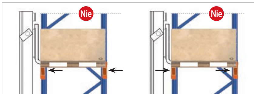
obr. 10 Obrat nosného trámu pri ťahaní alebo strkaní.
