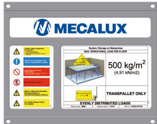
Príklad typového štítku
